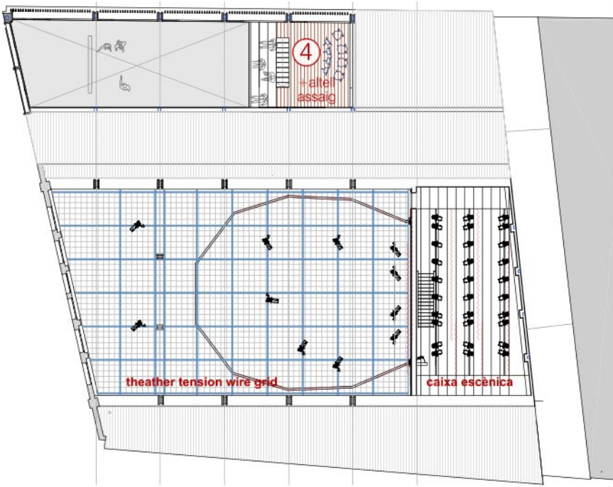
PLANTA TÈCNICA
