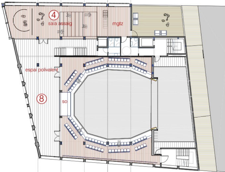
PLANTA SEGONA
