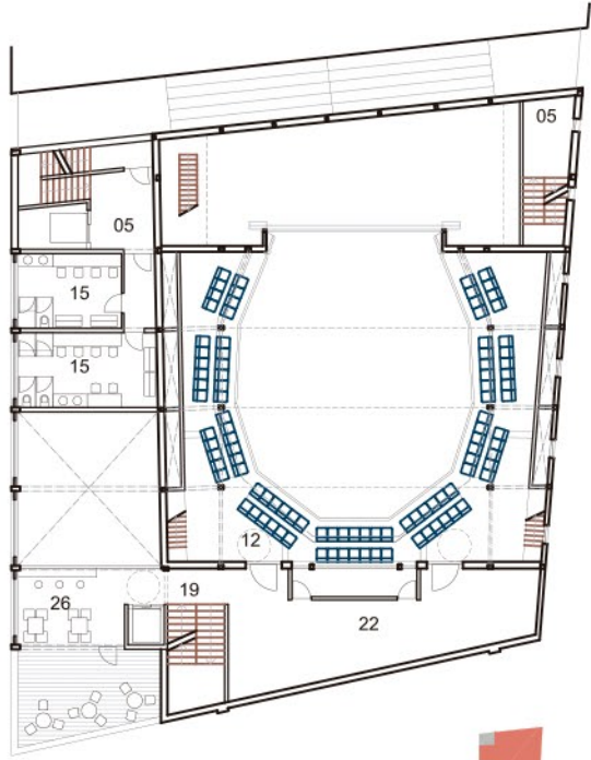
Planta primera
