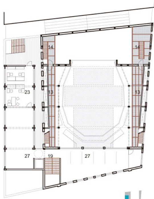
Planta segona
