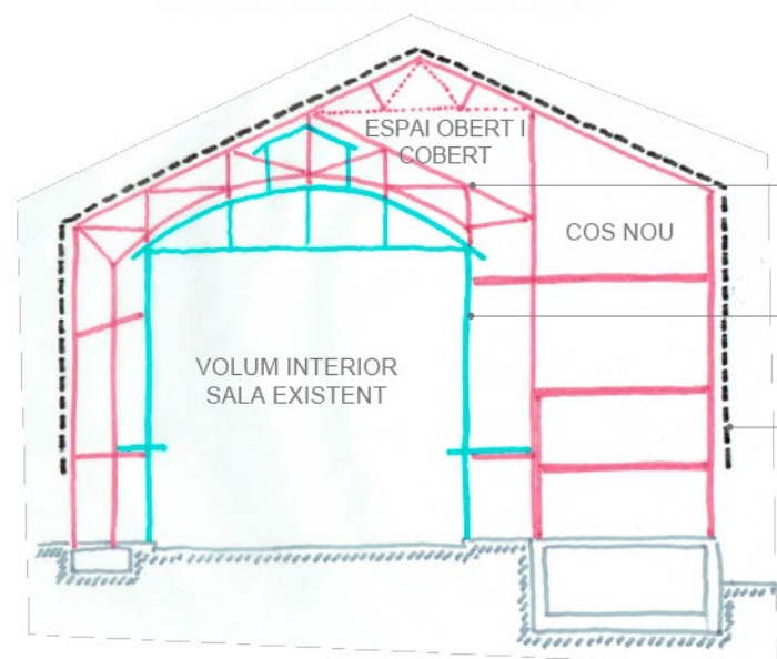
SECCIÓ TRANSVERSAL SALA e: 1/200
