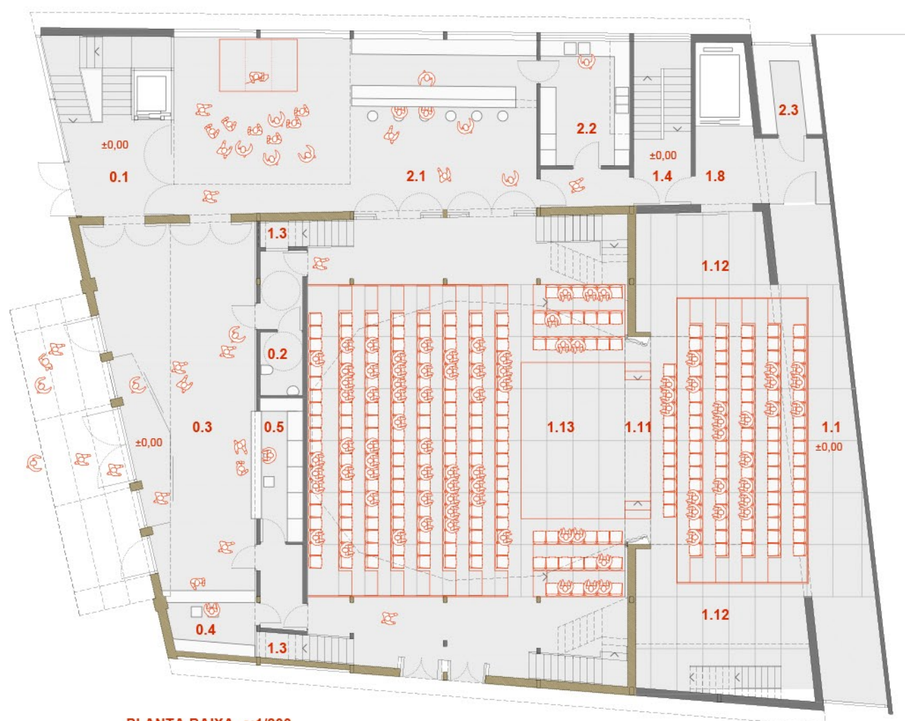
PLANTA BAIXA e: 1/200
