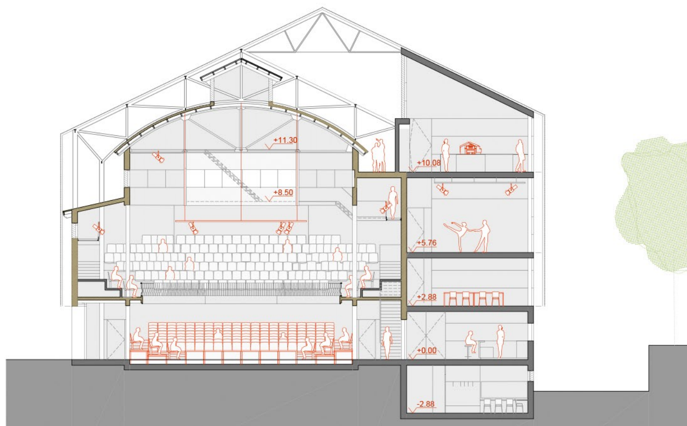
SECCIÓ TRANSVERSAL SALA e: 1/200
