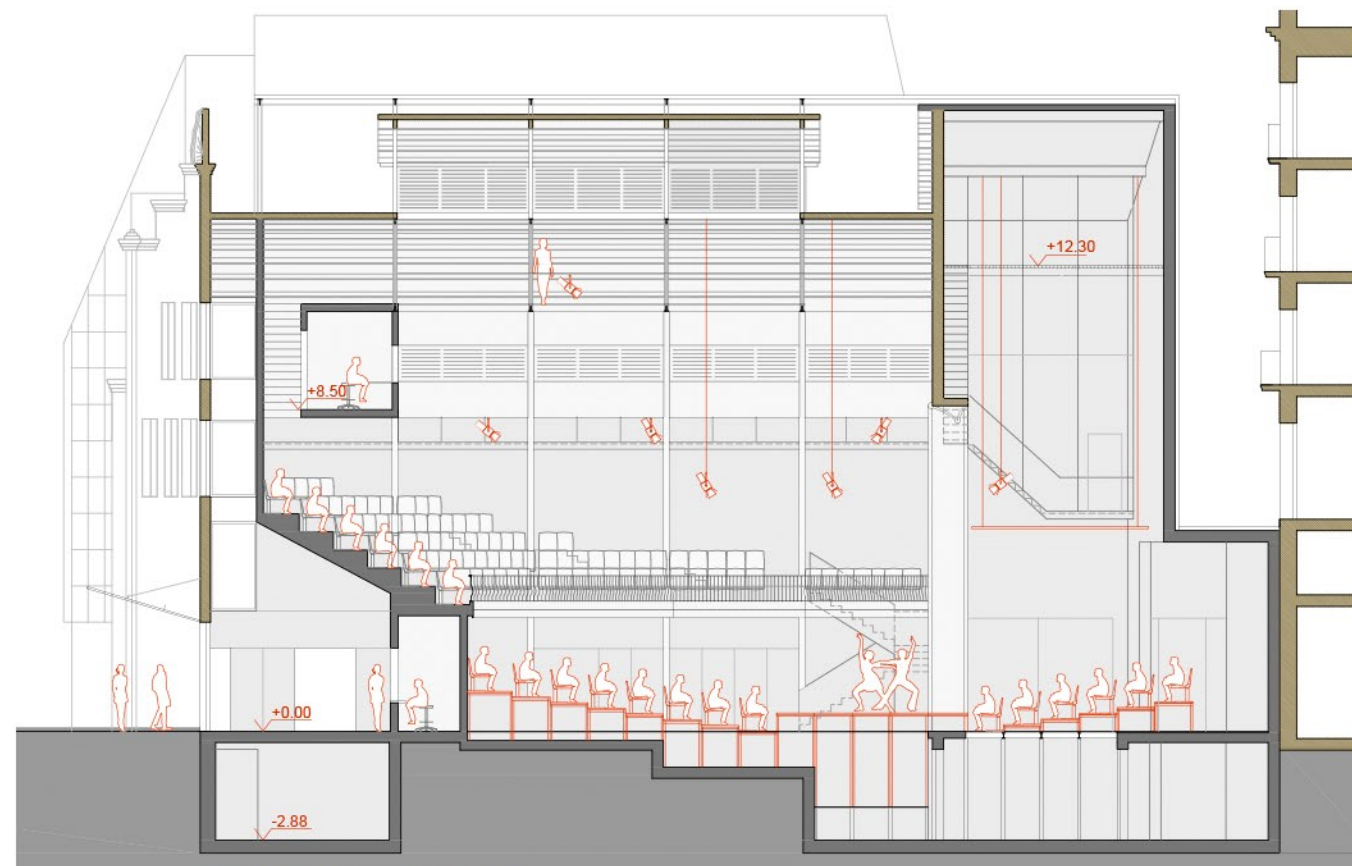
SECCIÓ LONGITUDINAL e: 1/200
