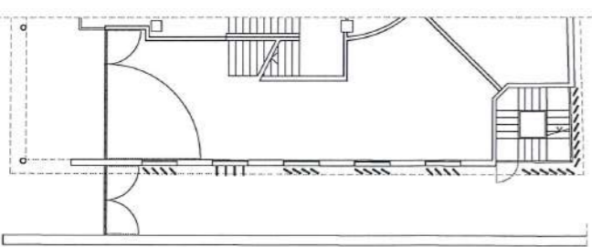
PLANTA BAIXA
