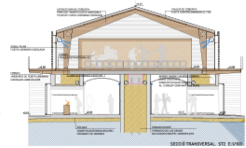
SECCIÓ TRANSVERSAL ST2. E.1/160
