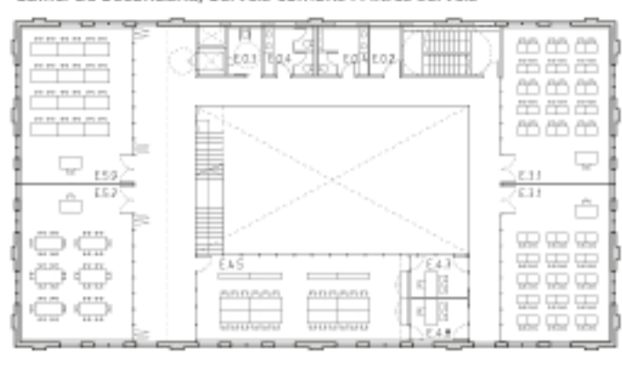
Planta Quarta E 1:400
