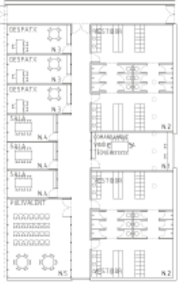
Planta Soterrani -1 E 1:400
