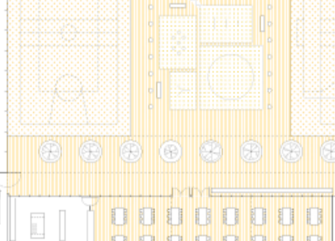
Planta Soterrani -1 E 1:400
