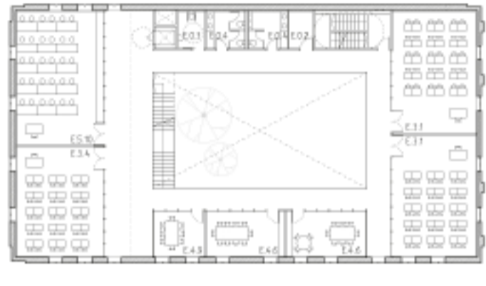
Planta Segona E 1:400
