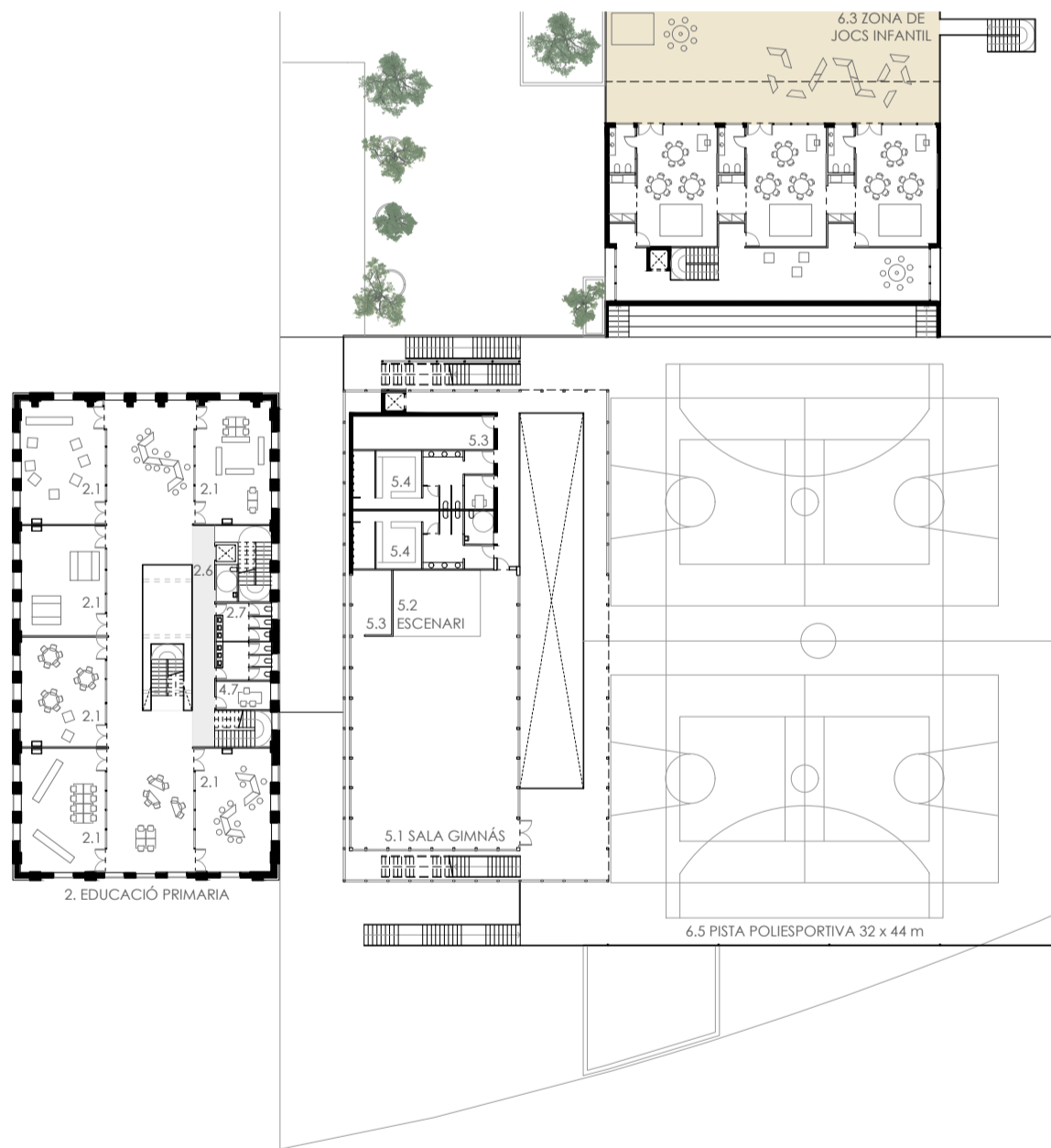
PLANTA 2 E:1/500 SUP. CONSTRUÏDA 1665m 2
