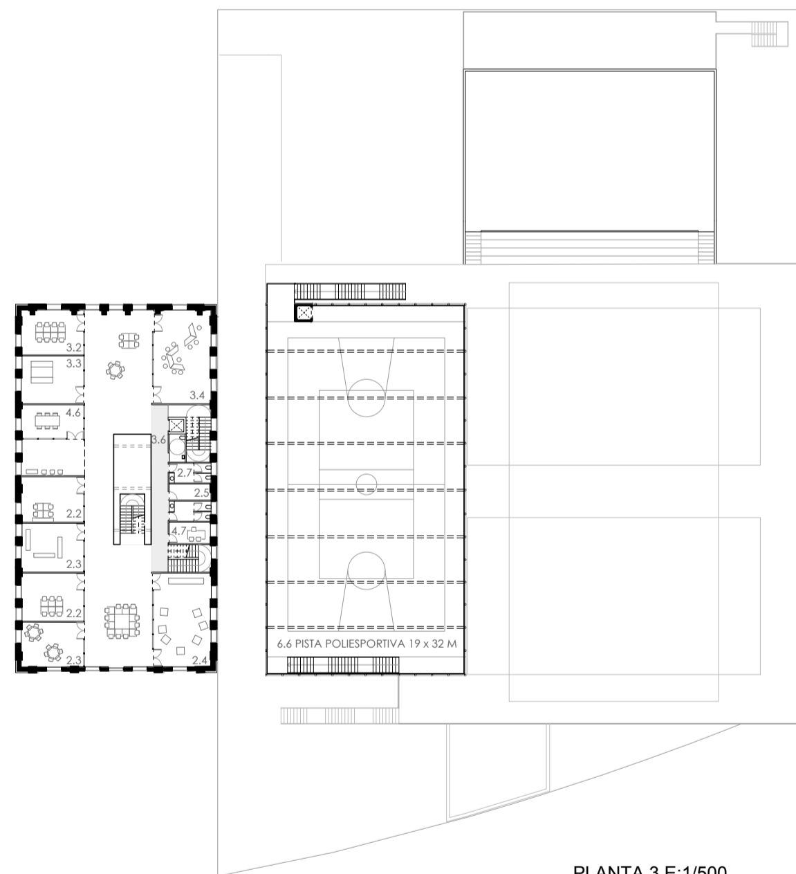
PLANTA 3 E:1/500 SUP. CONSTRUÏDA 1295m 2
