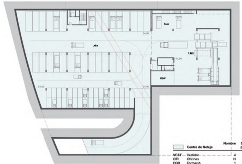
Planta Soterrani 1:500
