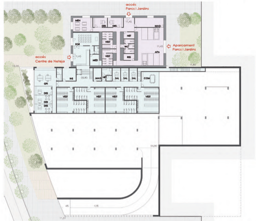
Planta Semisoterrani 1:500
