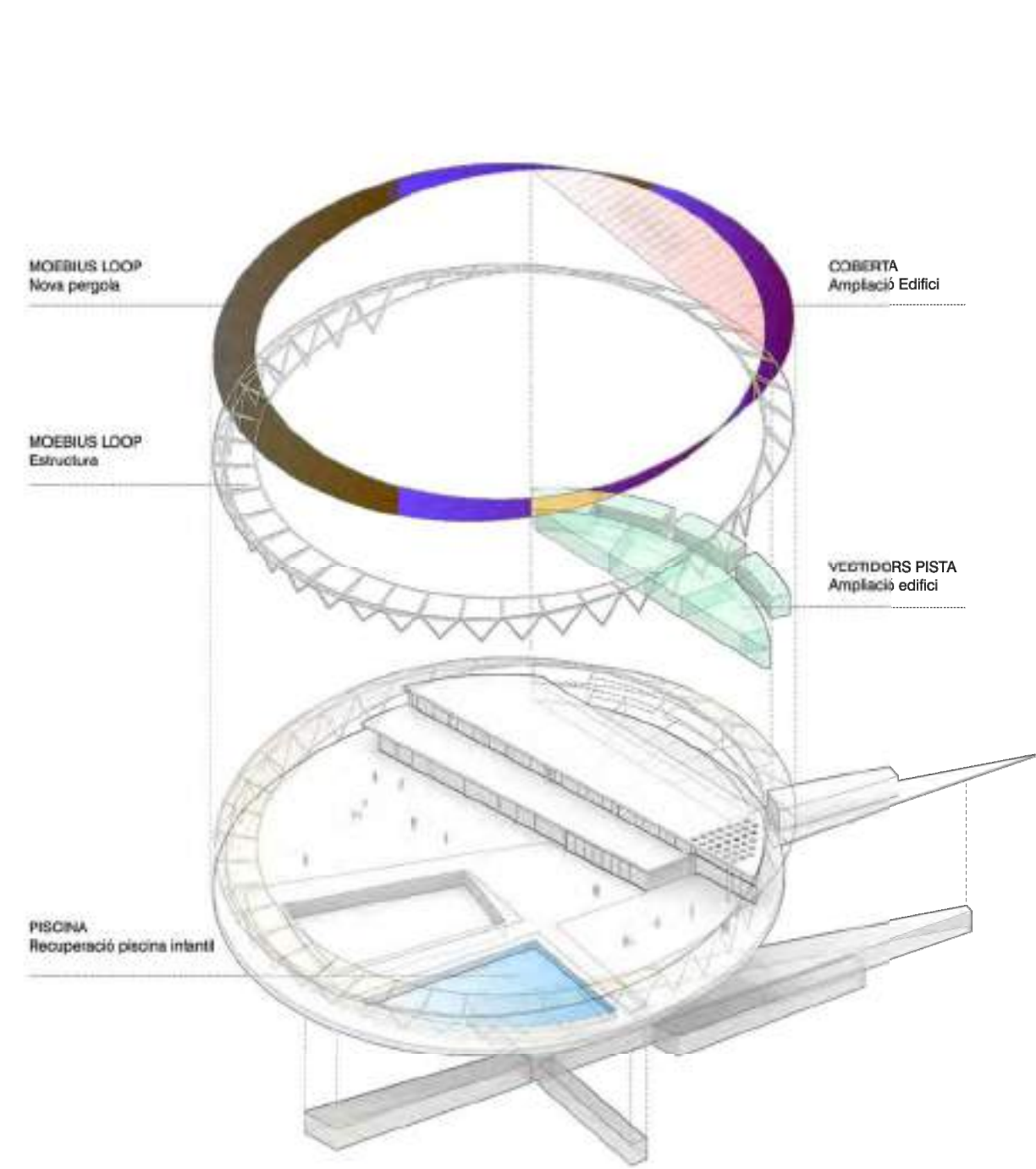
AXONOMETRIA AREA PISCINA
