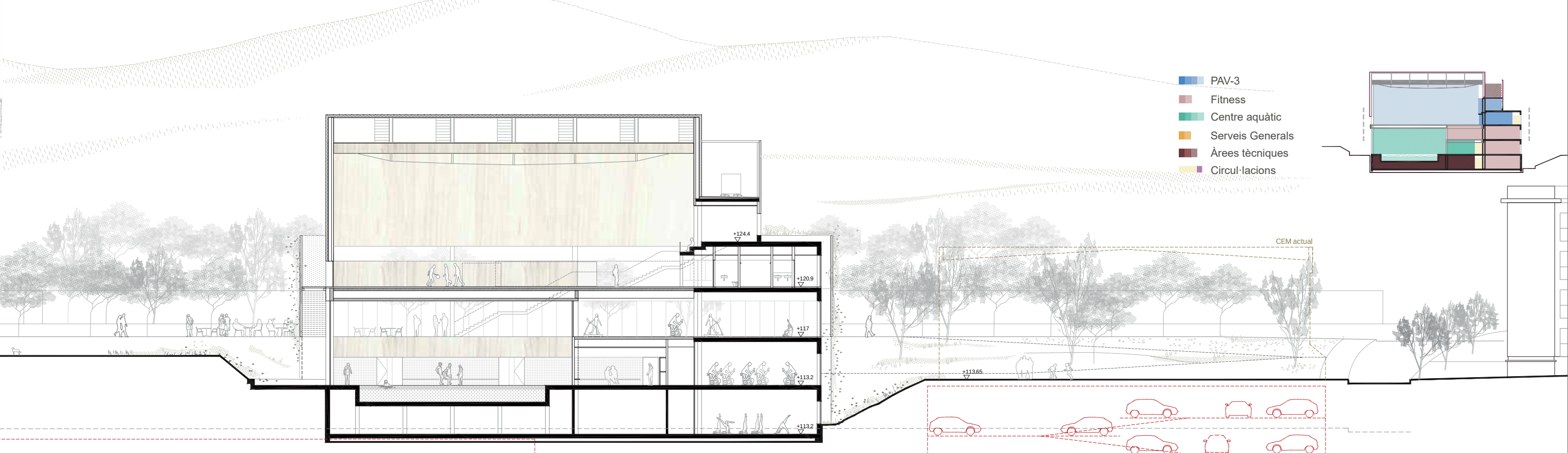
Secció Transversal
