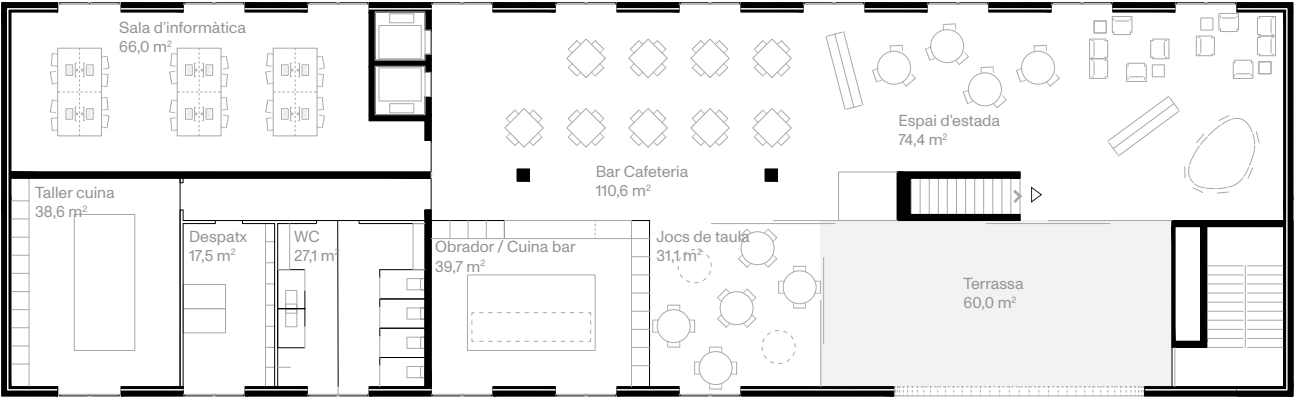
Planta Tercera. Casal de gent gran 1250
