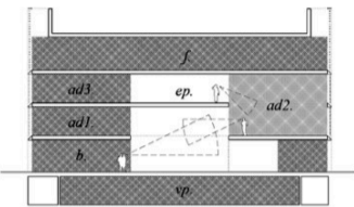
Secció Longitudinal (porxo) b. bar / t. terrassa / ep. vestidors de piscines / ad. activitats dirigides / f. sala de fitness / ep. espera prèvia
