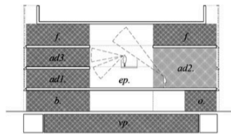
Secció Longitudinal (passera) b. bar / o. oficines i administració / ep. vestidors de piscines / ad. activitats dirigides / f. sala de fitness / ep. espera prèvia
