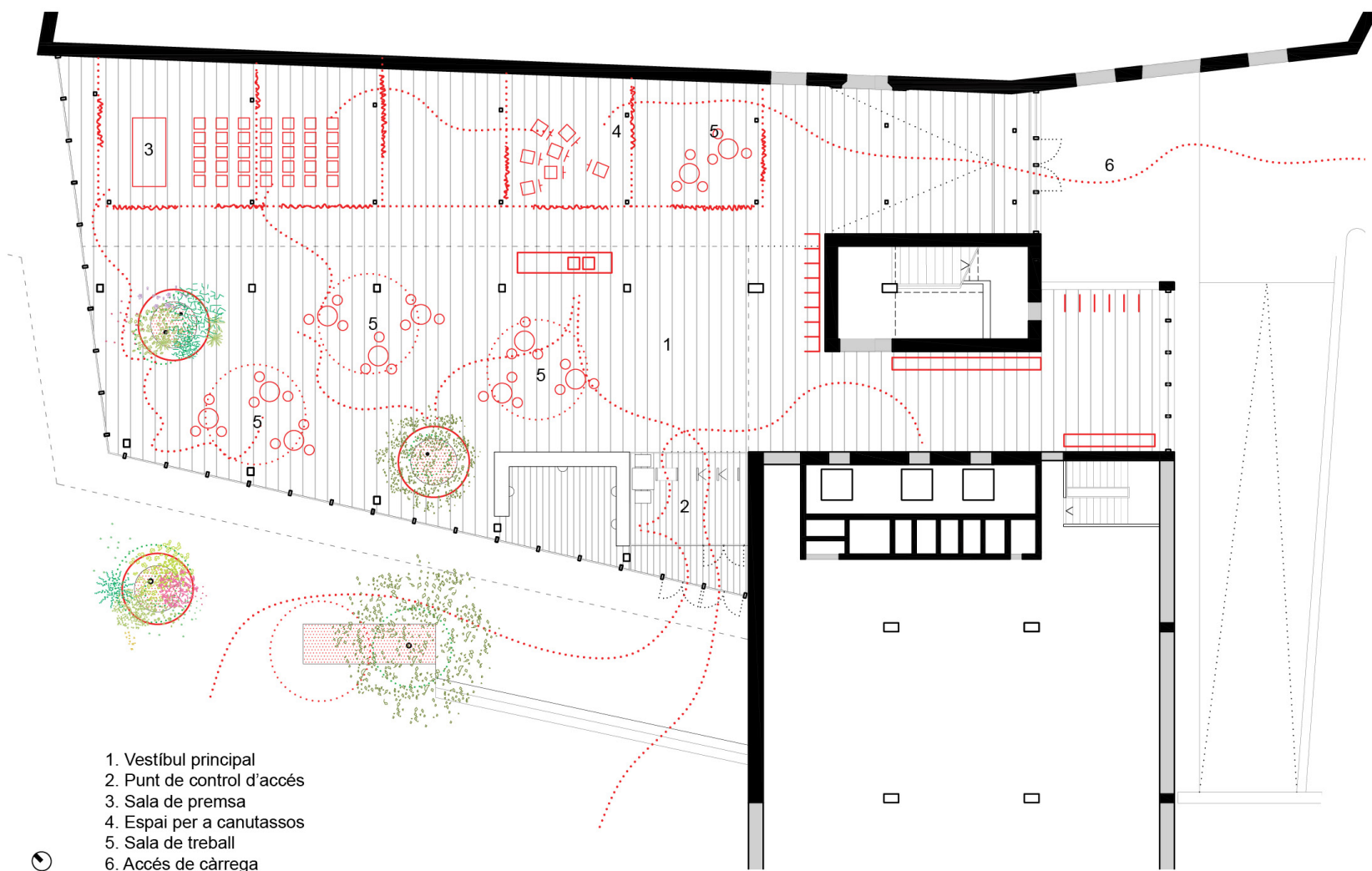
Planta Vestíbul 1:250
