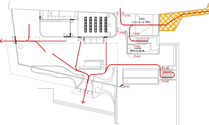
ESQUEMA EVACUACIÓ INCENDIS
