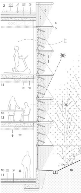
Detall Envolupant. 1:50
