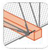
Detall 2 Unió cables viga
