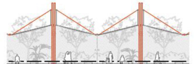
Alçat 1:250
