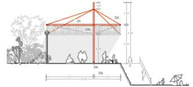
Secció 1:250
