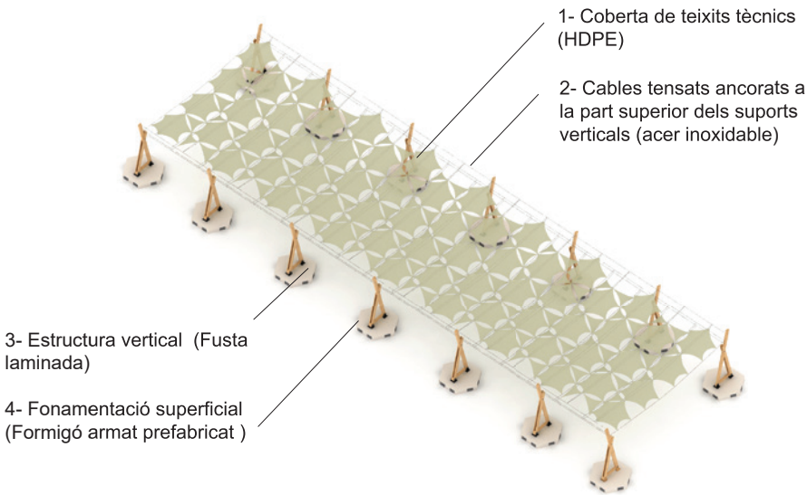
Axonometria de l'estructura d'ombra
