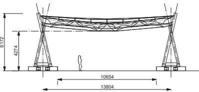
Secció transversal
