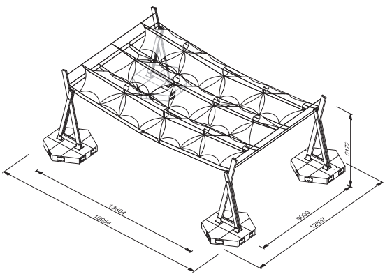
Axonometria del mòdul d'ombra
