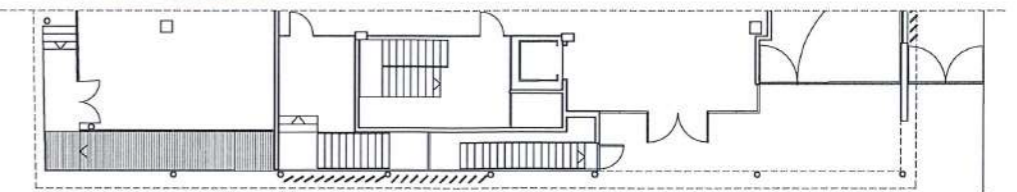
PLANTA BAIXA
