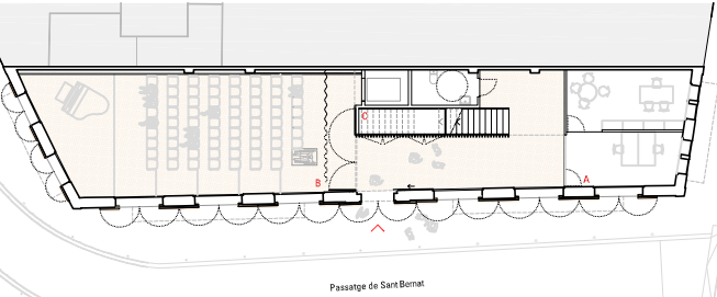
PLANTA BAIXA
