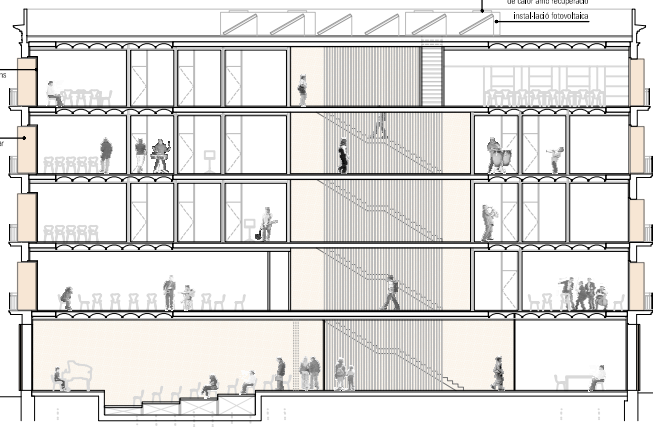
SECCIÓ LONGITUDINAL
