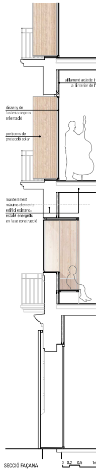
SECCIÓ FAÇANA
