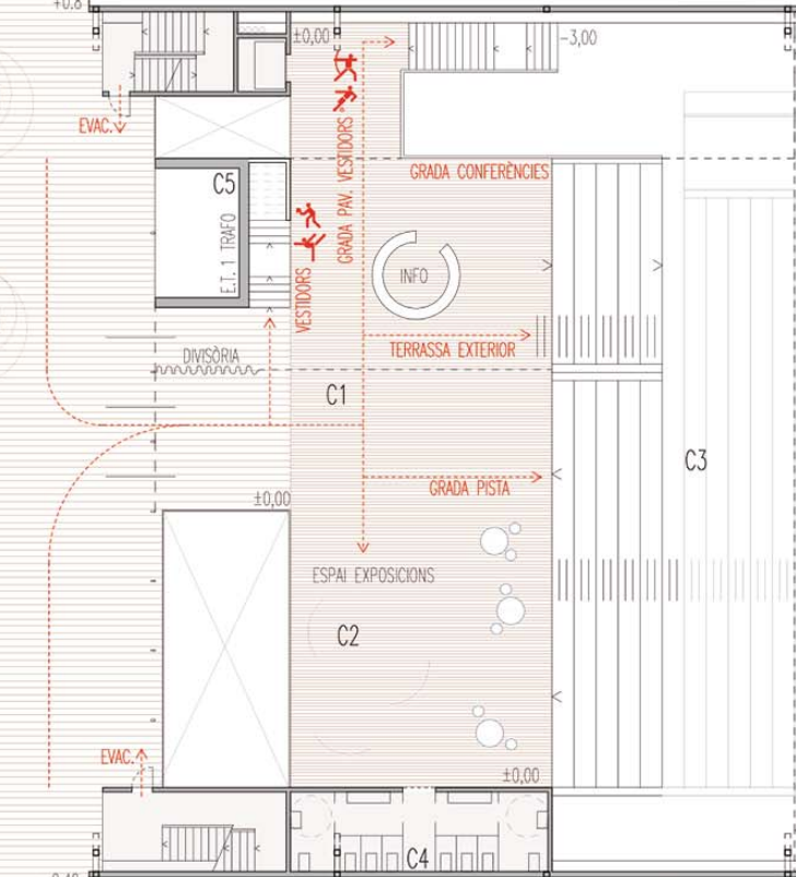
PLANTA COTA ±0,00 CARRER I PLAÇA COBERTA Serveis Comuns C1 Vestíbul-plaça i espai trobada 198 m 2 C2 Espai trobada 55 m 2 C3 Grada frontal pública 196 m 2 C4 Serveis Generals 30 m 2 C5 Estació Transformadora 21 m 2 nuclis i circulacions 89 m 2 e 1:300
