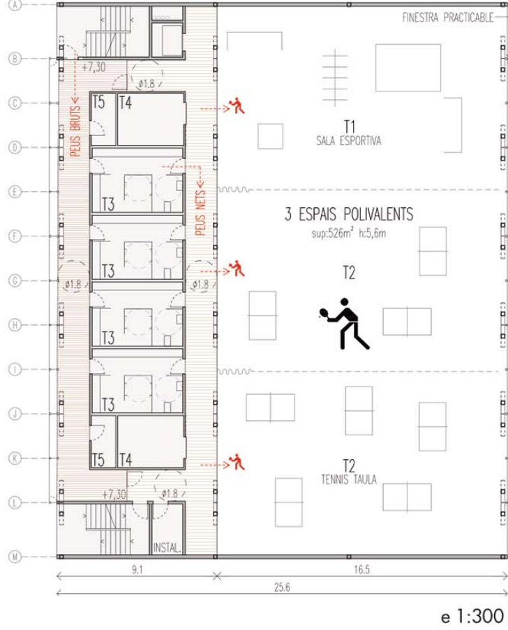
PLANTA COTA +7,30 ← TENNIS TAULA I SALA ESPORTIVA Tennis taula i s. esportiva T1 Sala Esportiva 171 m 2 T2 Sala de Tennis Taula 342 m 2 T3 Vestidors (4ut) 83 m 2 T4 Magatzem (2ut) 30 m 2 T5 Neteja 7 m 2 nuclis i circulacions 155 m 2 instal·lacions 5 m 2 → PLANTA COTA +10,15 ALTELL VESTUARIS GIMNÀSIA Gimnàstica Artística G1 Vestidors (4ut) 83 m 2 G2 Neteja 30 m 2 G3 Magatzem 7 m 2 nuclis i circulacions 176 m 2 instal·lacions 5 m 2 e 1:300
