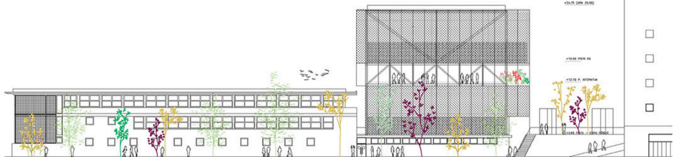
Alçat Carrer Constança E/1:300
