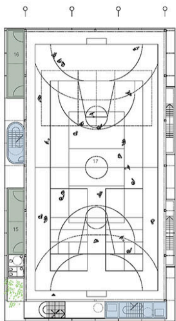
P3 Planta pista 2 + 15.50 m E/1:300
