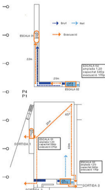
PB Recorregut Peus Bruts Peus Nets
