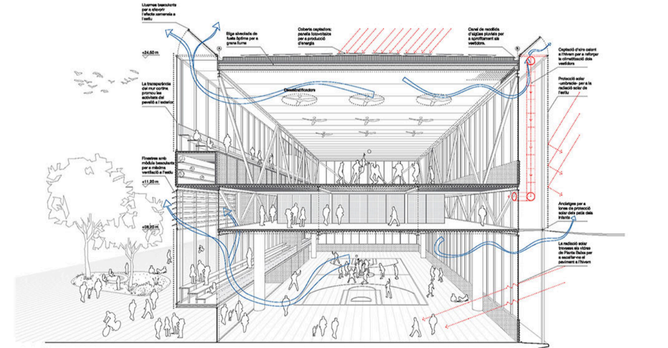
Secció constructiva climàtica
